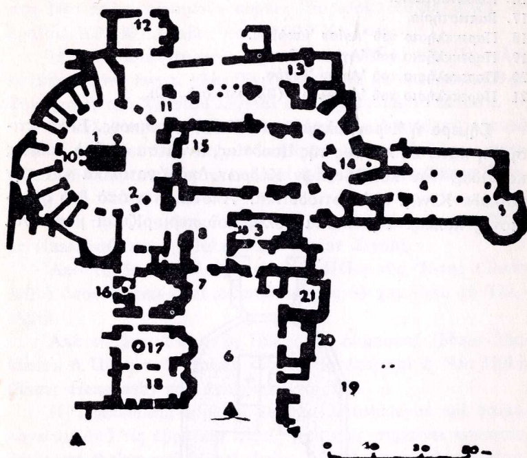
Εἰκ. 7. — Ἱερουσαλήμ. Κάτοψη τοῦ ναοῦ τοῦ Ἁγίου Τάφου. (AVRAHAM LEWENSOHN, Israel Tourguide, Tel Aviv 1978), p. 271).
