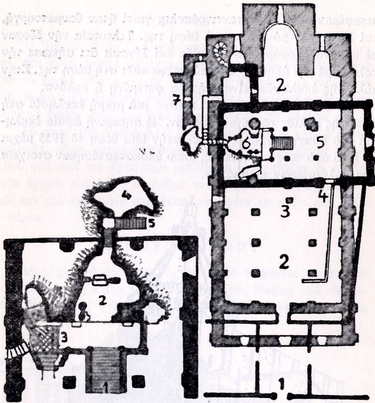
Είκ. 3. — Ναζαρέτ. Ὁ ναὸς τοῦ Εὐαγγελισμοῦ. Κάτοψη.
